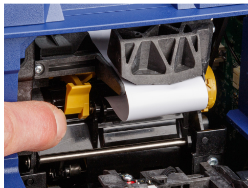
Abziehvorrichtung geschlossen
