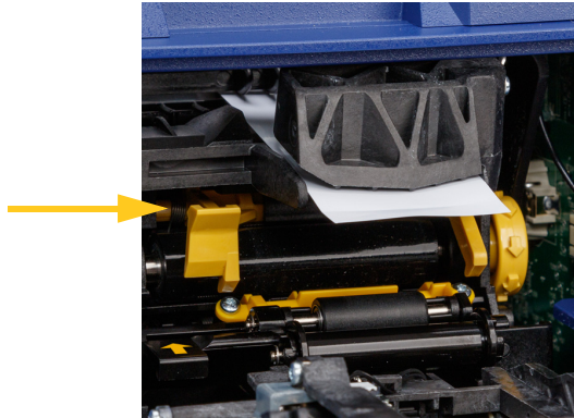
Abziehvorrichtung geöffnet
