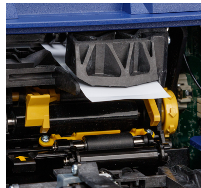
Abziehvorrichtung geöffnet
