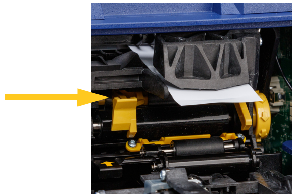
дверца механизма отделения открыта
