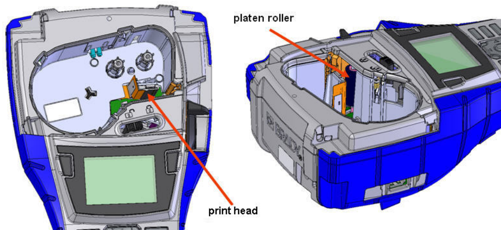
Figur 39 • Printhoved og valserulle i kassettebås
