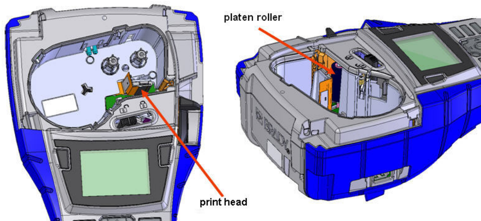
Рисунок 39. Печатающая головка и валик в отсеке для картриджа
