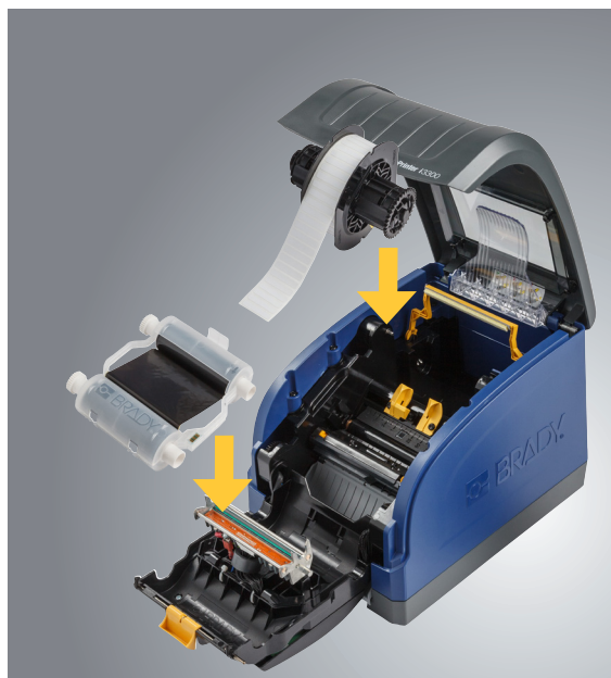
Chargement facile par le dessus
