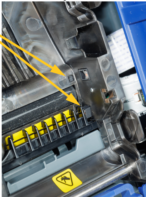
Figur 2-2. Posisjonen til forkanten av etikettmaterialet.
